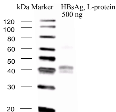
Fig. 2 HBsAg, Lタンパク質のウエスタン・ブロッティング
